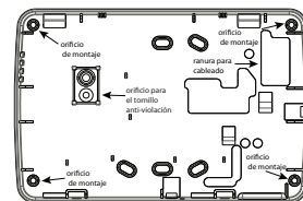
Figura 2 – Montaje de la placa de apoyo
